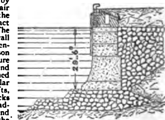
FIG. 15.—Caracciolo Jetty Quay Wall, Genoa.
